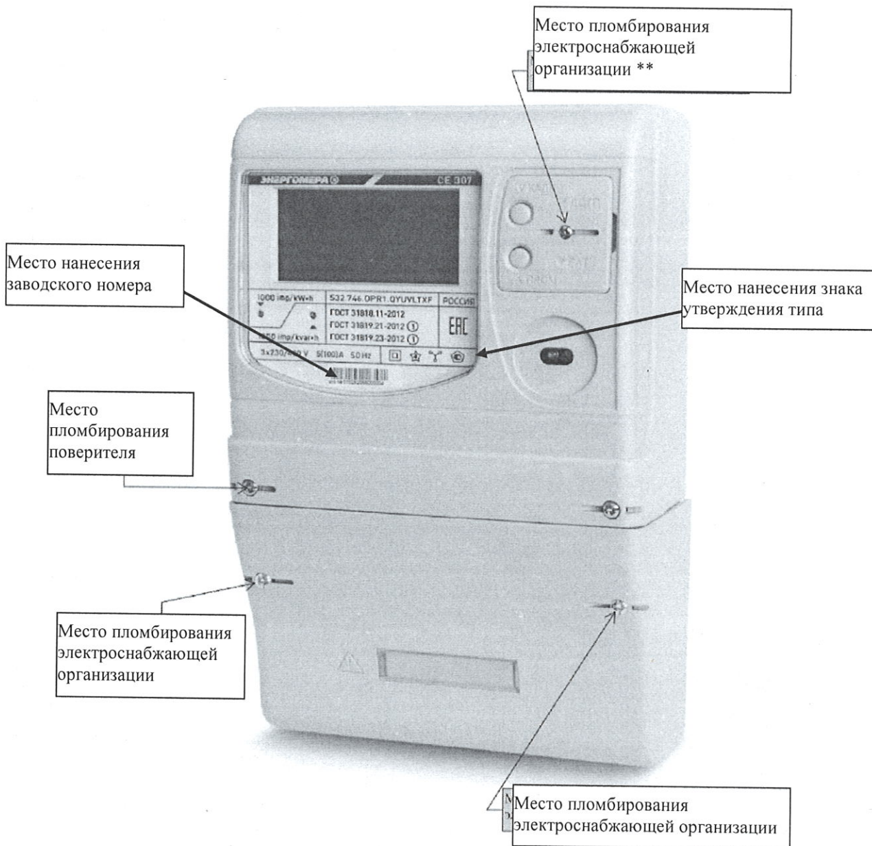
Рисунок 9 – Общий вид счетчика CE307 S32
